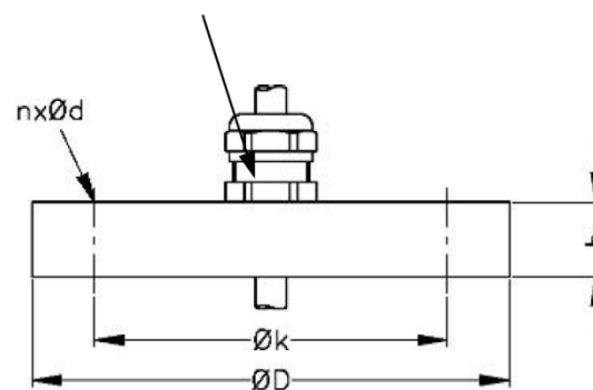
Кабельный ввод M16x1.5 под кабель Ø 4..11 мм
